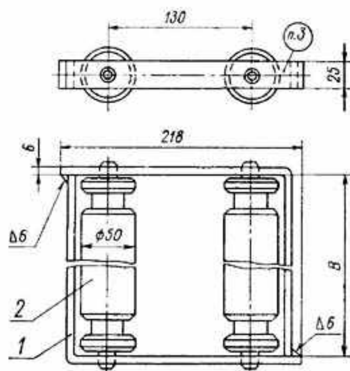
1 — угольник; 2 — направляющий
